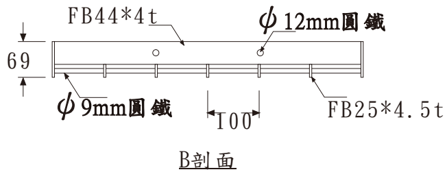
熱浸鍍鋅化妝蓋板尺寸
